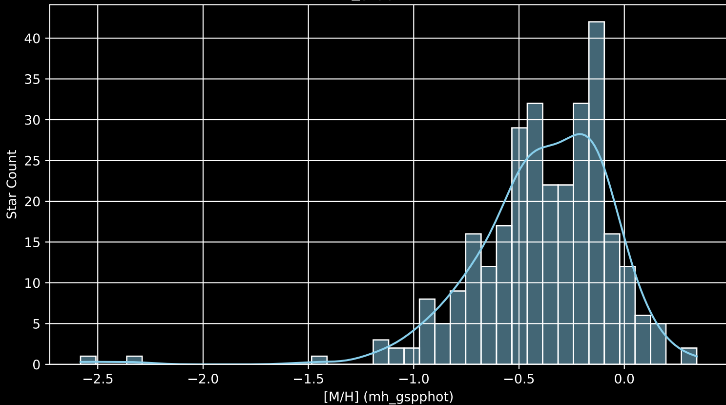
GALAH DR4 Field: [475] [M/H] (mh_gspphot) (n= 297)
