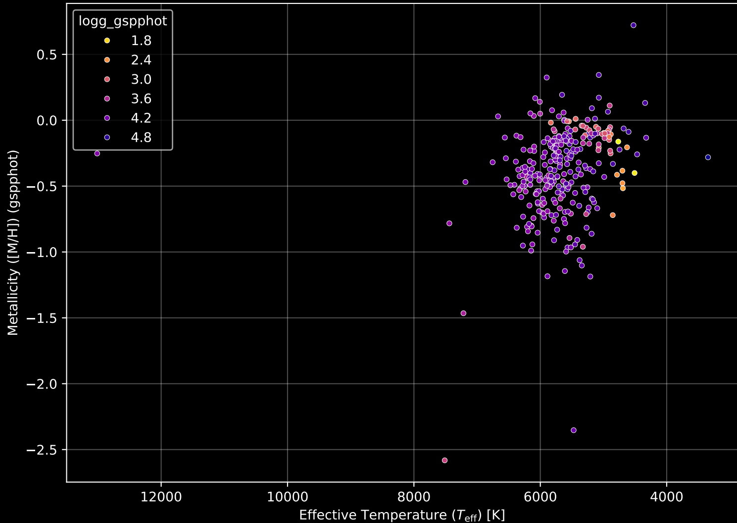
GALAH DR4 Field: [475] Stellar Population Parameters (n= 298)
