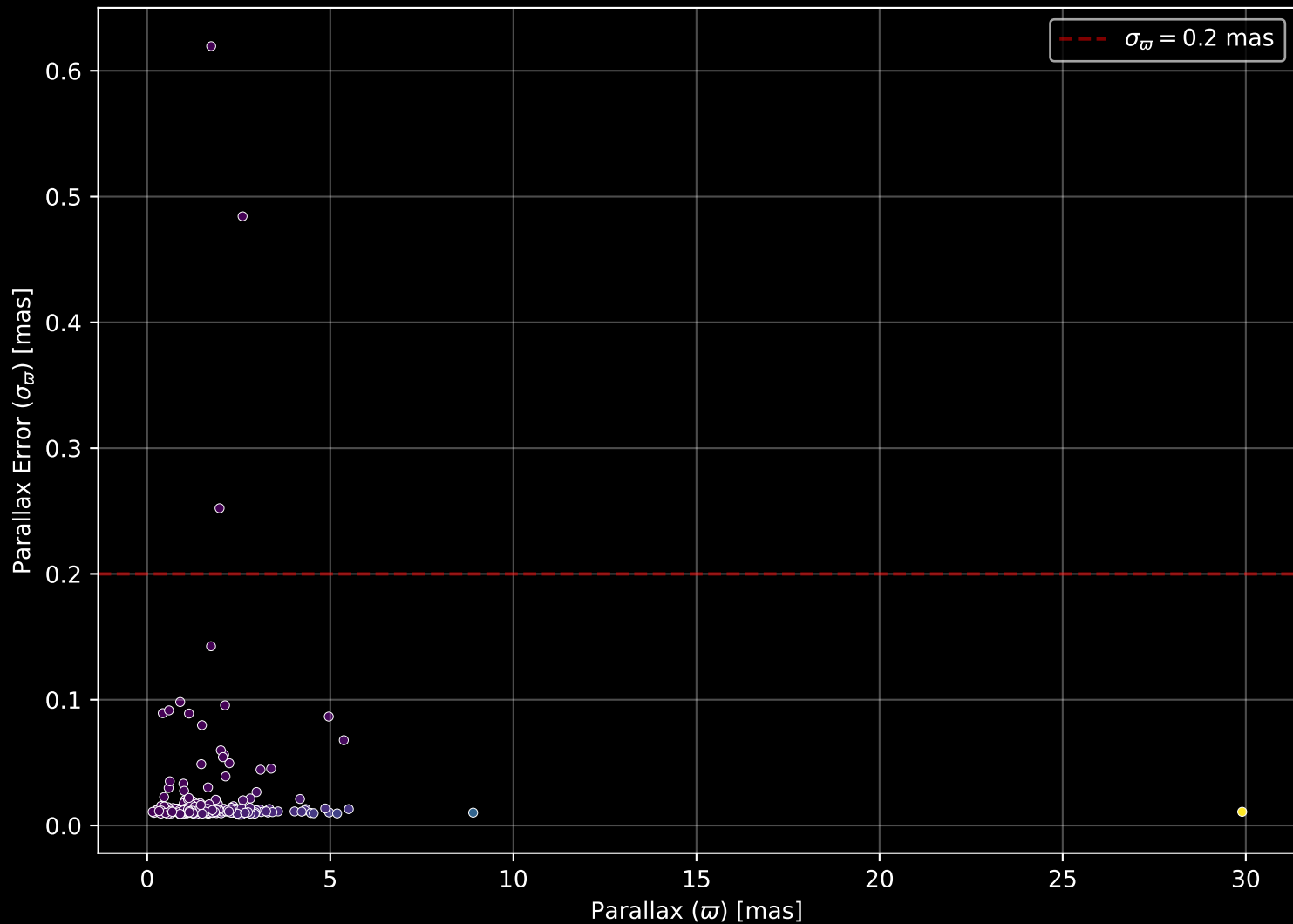
GALAH DR4 Field: [475] Parallax Quality (n= 298)
